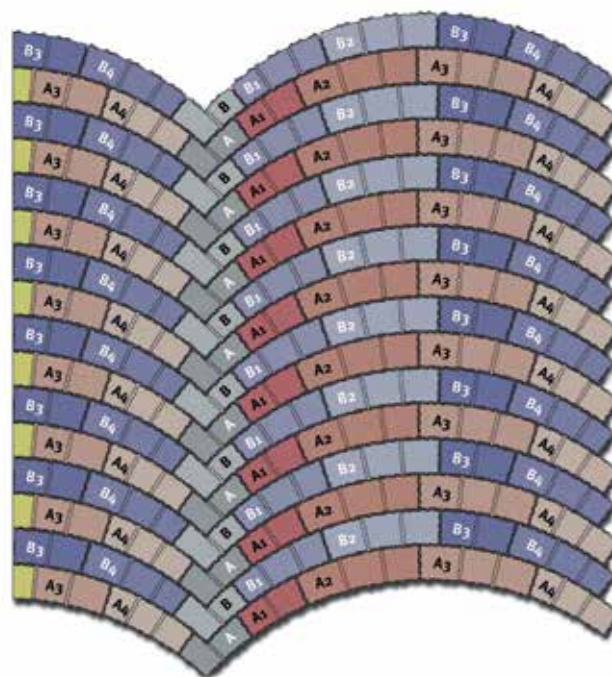
Fig. 4: Închiderea pe margine Din pavajul de margine A3 este tăiat, iar la pavajul B3 sunt tăiate doar elementele de îmbinare.
